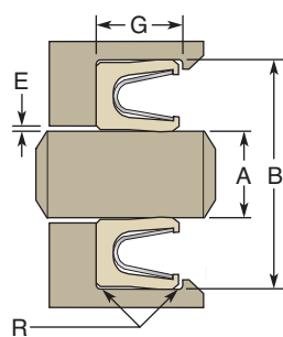
Rod Seal
