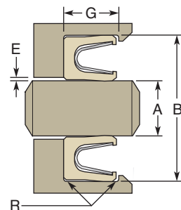
Rod Seal
