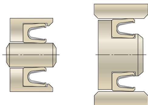
Rod Gland
