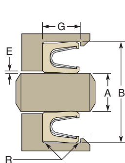
Rod Seal
